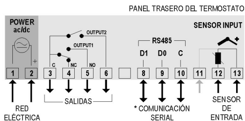
Figura 01 – Conexiones mostradas en la etiqueta del termostato
