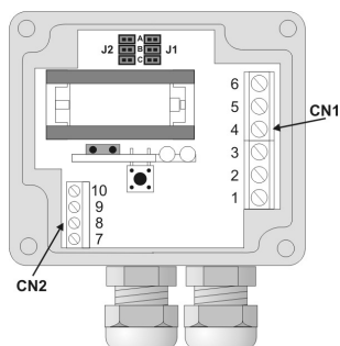
Figura 08 – Versión IP65, vista interna de las conexiones
