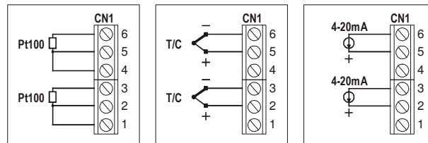
Figura 09 – Conexiones del señal de entrada
