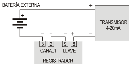
Figura 10 – Ejemplo de utilización del accionamiento externo
