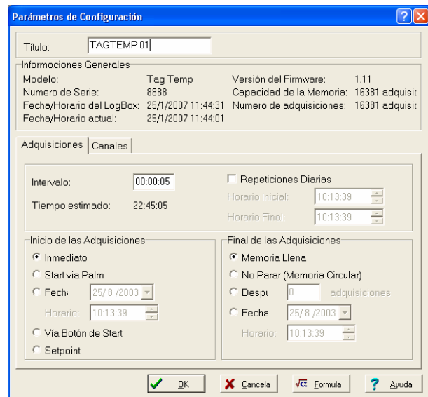
Figura 07 – Parámetros de configuración de los canales de entrada
