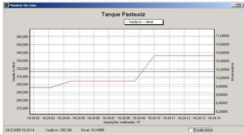
Figura 14 – Gráfico de monitorización on-line
