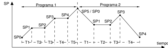
Figura 12 - Ejemplo de programa 1 e 2 "linkados" (interconectados)
