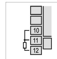
Figura 4 - Conexión de Pt100 a 3 hilos
