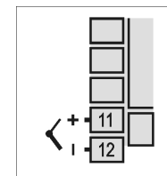
Figura 3 - Conexión de termocupla (T/C)
