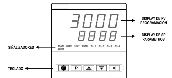
Figura 1 - Identificación de las partes del panel frontal
