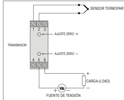
Figura 5 – Conexiones eléctricas del transmisor – Termocupla
