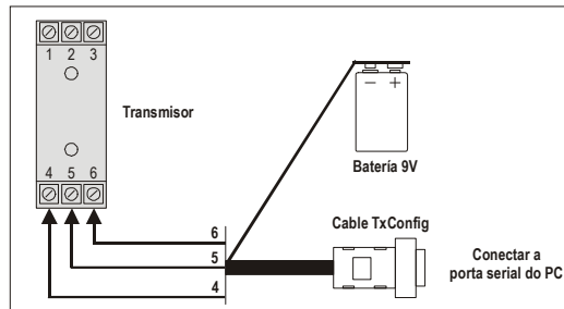
Figura 1 – Conexión del cable convertidor al transmisor
