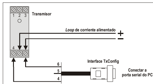
Figura 02 – Conexión del Cable TxConfig – Alimentación pelo loop
