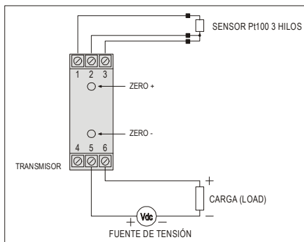
Figura 04 – Conexiones eléctricas del transmisor – Pt100
