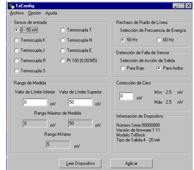
Figura 02 – Pantalla principal del software TxConfig
