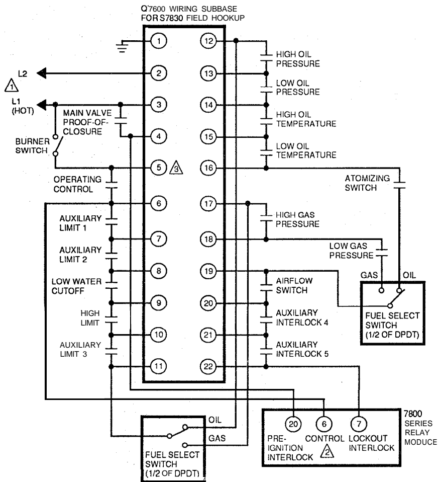
Fig. 3—S7830 wiring hookup.
