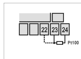
Figura 4 - Conexión de Pt100 a 3 hilos
