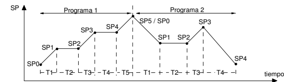
Figura 12 - Ejemplo de programa 1 e 2 "linkados" (interconectados)
