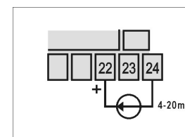
Figura 5 - Conexión de corriente
