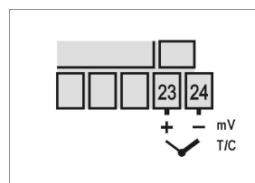
Figura 3 - Conexión de termocupla (T/C)
