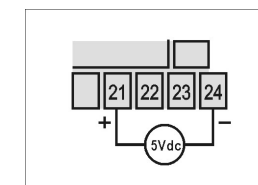
Figura 6 - Conexión de Tensión 0 – 5Vdc
