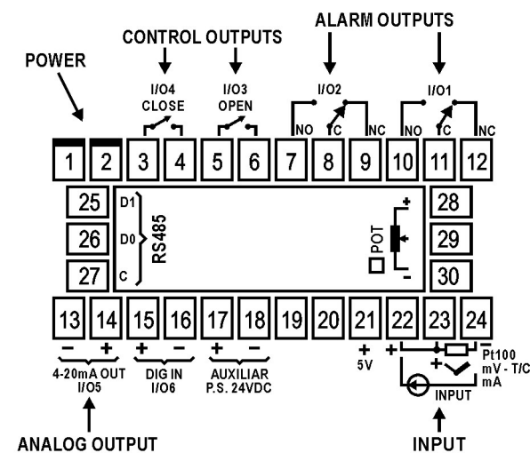
Figura 2 - Conexiones del panel trasero.
