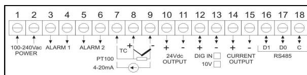
Figura 3 - Conexiones del panel trasero
