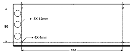
Figura 2 - Fijación del indicador al panel de instrumentación
