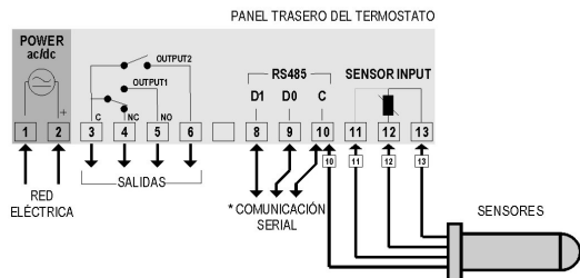
Figura 01 – Conexiones mostradas en la etiqueta del controlador
